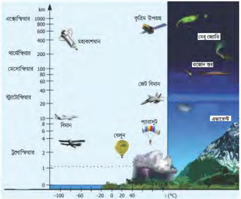
বায়ুমণ্ডলের স্তরবিন্যাস
